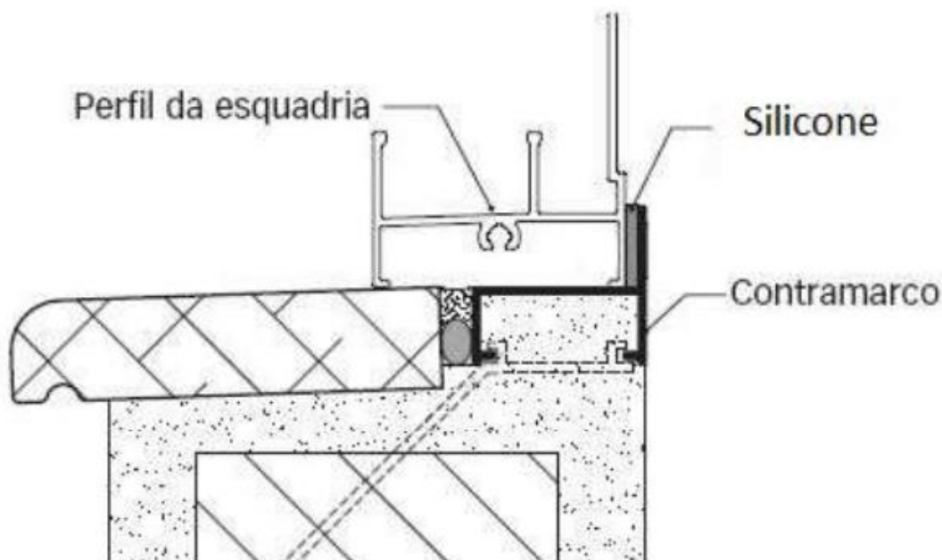
Figura 3 - Detalhe de instalação das esquadrias janelas com perfil cadeirinha
