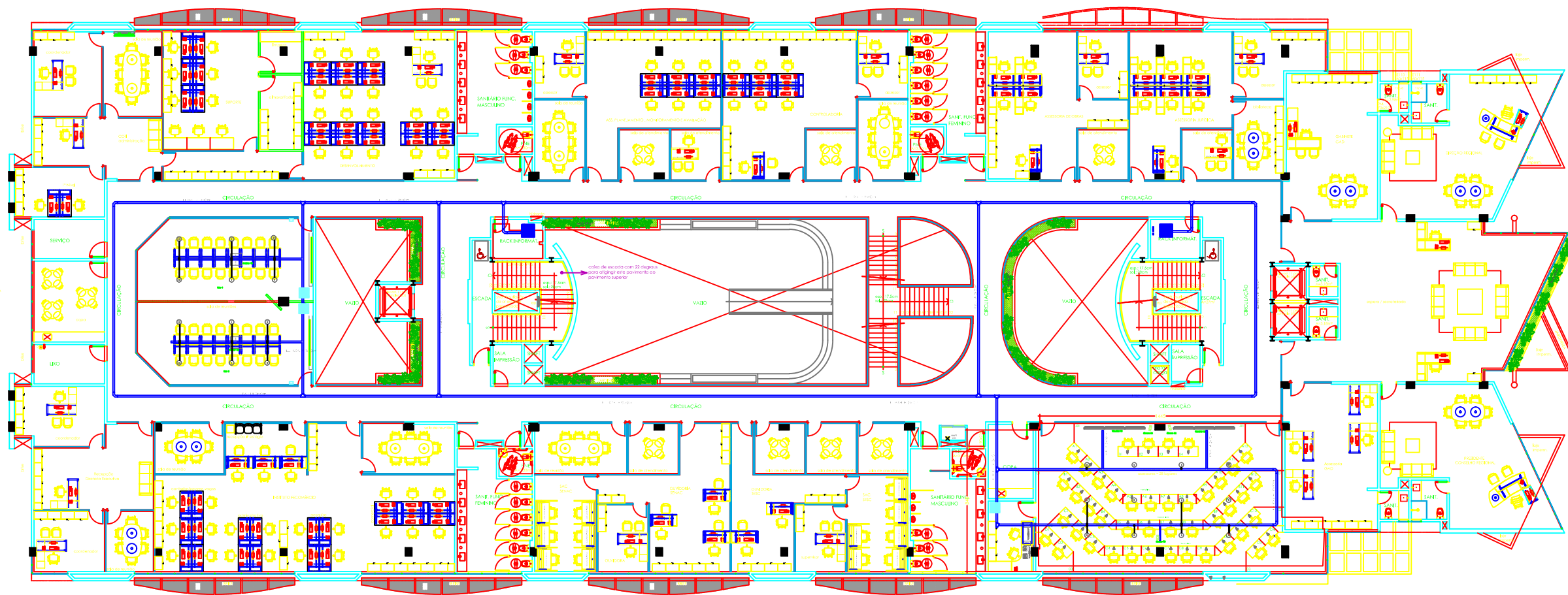
PLANTA BAIXA QUARTO PAVIMENTO SESC SEDE - esc.:1/100
